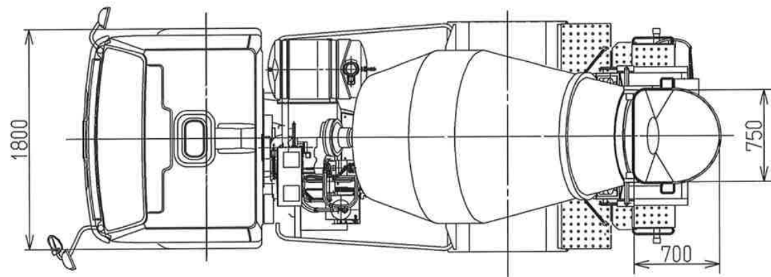
ミキサアジテータトラック外観図
